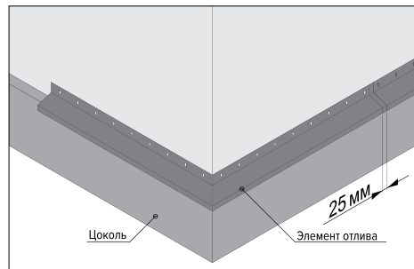
Рис. 3.1. Установка цокольного отлива
