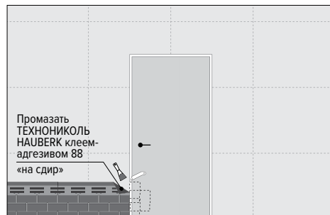
Рис. 7.1. Монтаж фасадной плитки вокруг дверных проемов
